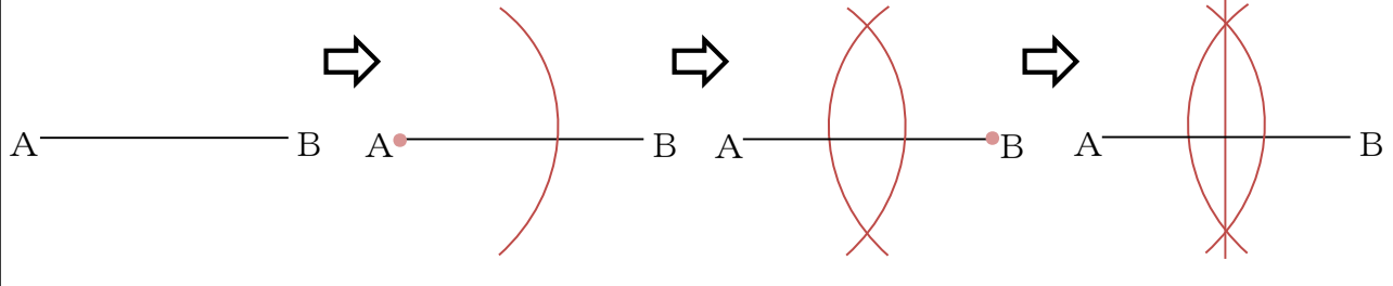
線分 AB の垂直二等分線の作図
