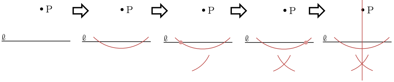
直線 l 上にない点 P を通る垂線の作図①
