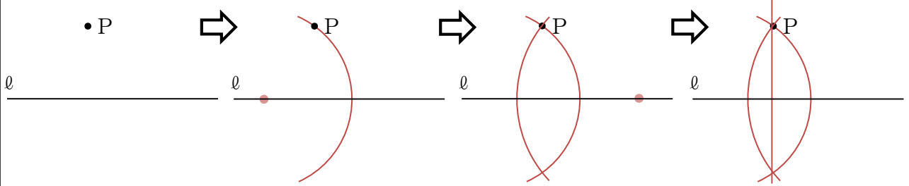
直線 l 上にない点 P を通る垂線の作図②
