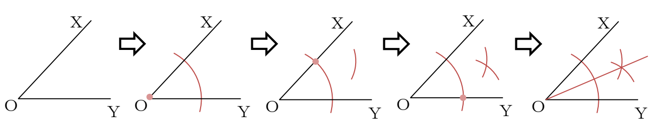
角の二等分線の作図
