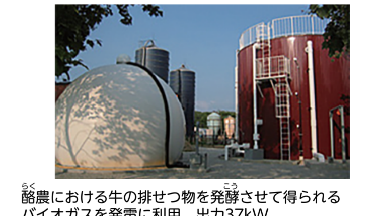
酪農における牛の排せつ物を発酵させて得られるバイオガスを発電に利用。出力37kW
