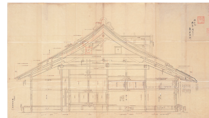
重要文化財「御本丸御座間二拾分ノ一妻建地割」
