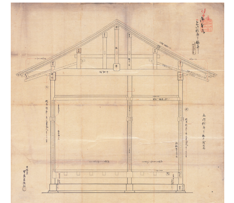
重要文化財「御本丸上御鈴廊下矩計」
